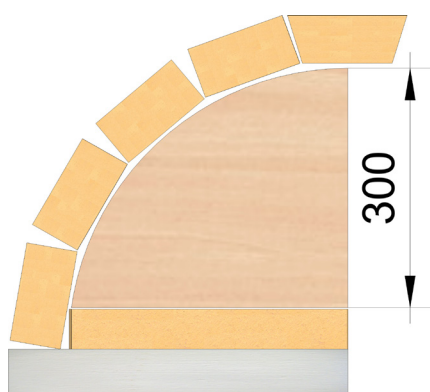
Anordnung Kuppelwand
