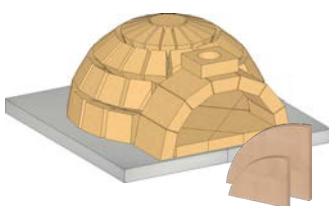
Schamottesatz und Schablonen
